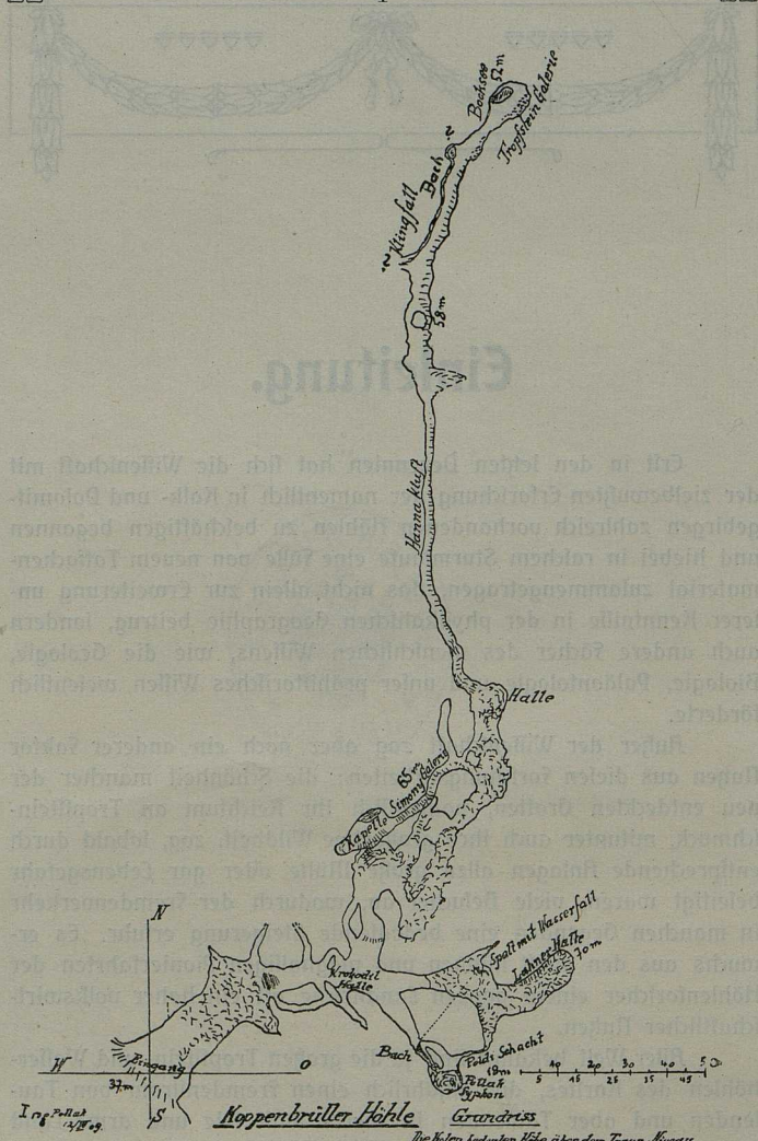
Plan der Koppentrillerhöhle.
