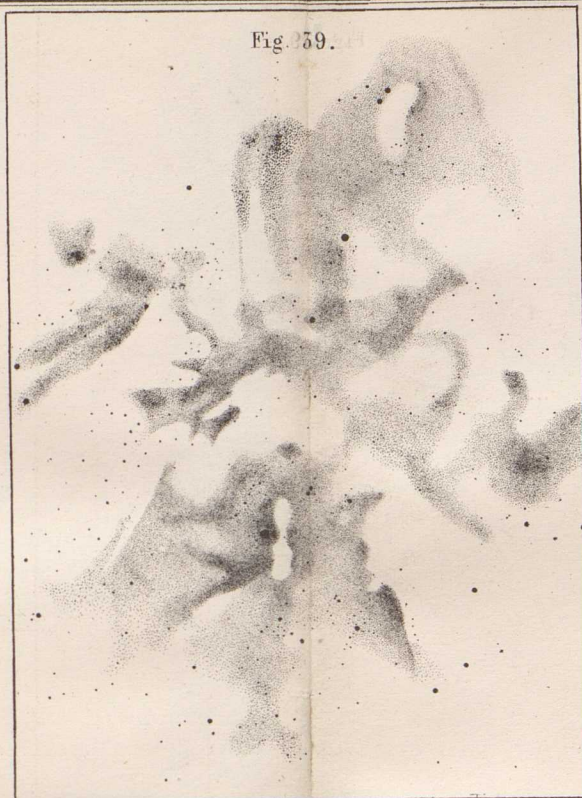
Nebel bei η Argus.
