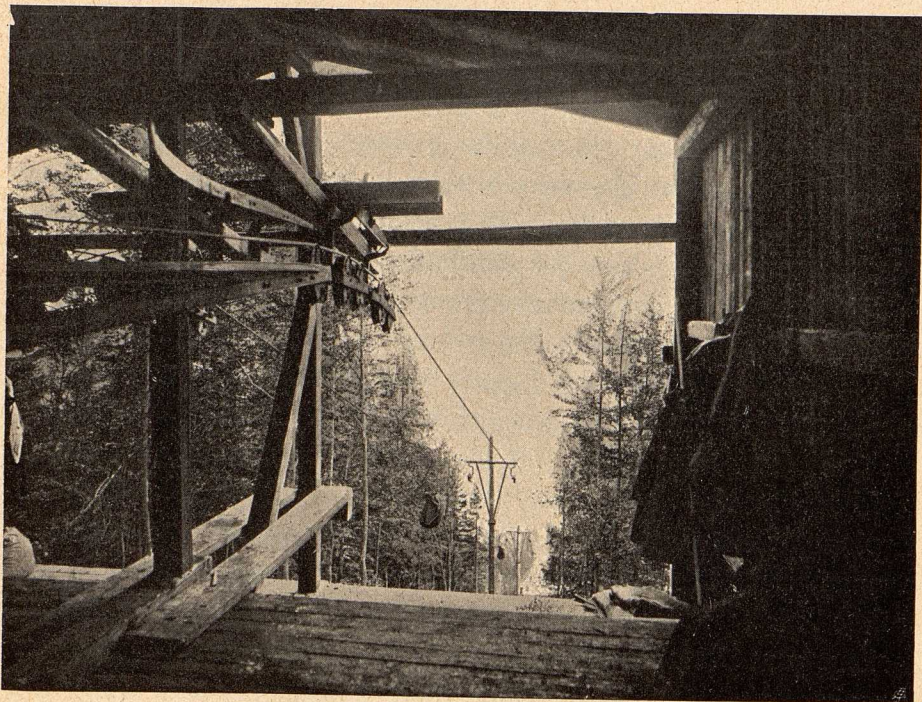
Bild 21. Photo Findeis: Militärische Drahtseilbahn. Endstation.
