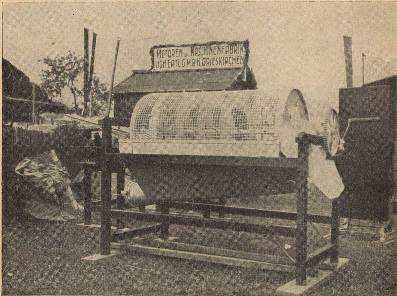
Gemeinschaftliche Verwendung landwirtschaftlicher Maschinen und Geräte in bäuerlichen Betrieben: Kartoffelwaschmaschine, Fabrikat Ertl, Grieskirchen. Für die gemeinschaftliche Durchführung der Kartoffeleinsäuerung konstruiert.
