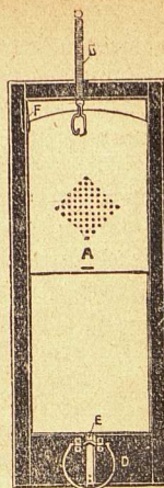
A. Metalltür. B. Zugfeder. C. Krippe. D. Krippenhalter. E. Flachfeder. F. Klemmfeder.
