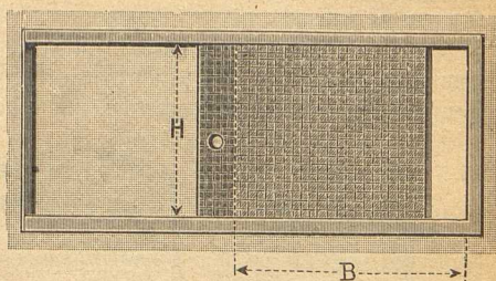
Drahtglas-Schiebfenster.
