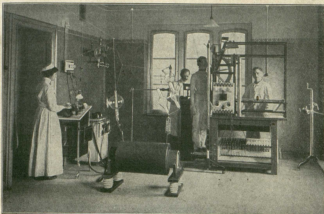
Fig. 14. Röntgenkinematograph. Aufnahme eines Geschosses im Herzen
