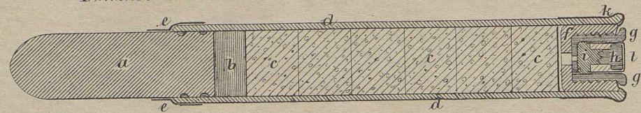
Fig. 4. Durchschnitt der Patrone in natürlicher Grösse.
