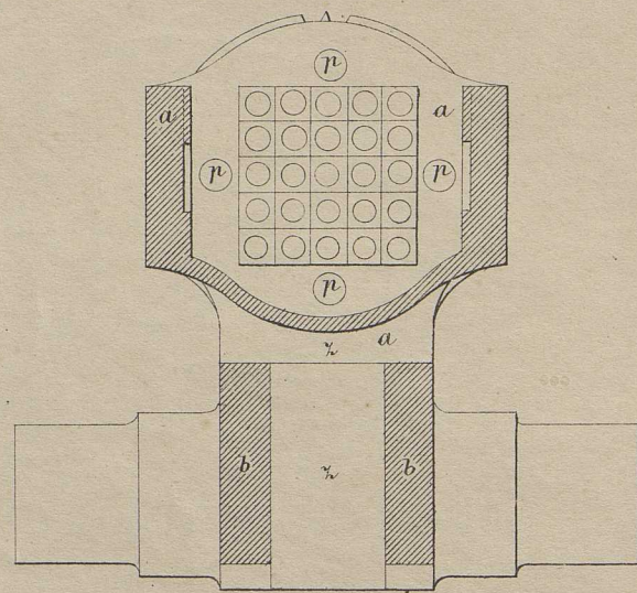
Fig. 4. Durchschnitt der Patrone in natürlicher Grösse.
