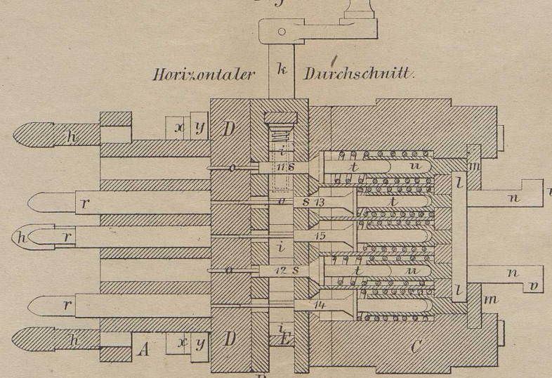
Fig. 10. Zündbohrer, 1/2 nat. Gr.
