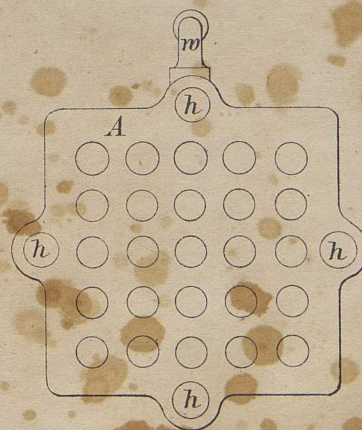
Fig. 5. Vorderansicht der Ladebüchse.
