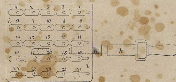
Fig. 5. Vorderansicht der Ladebüchse.
