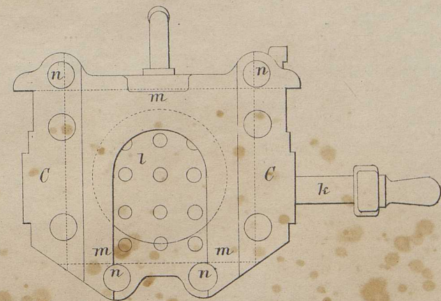
Fig. 8. Hintere Ansicht der Federbüchse.
