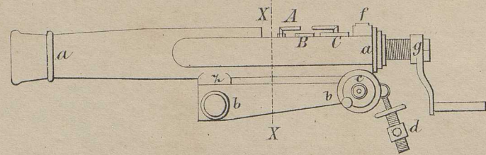
Fig. 2. Obere Ansicht 1:20
