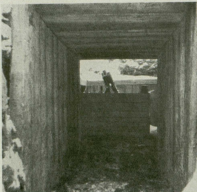
Eingebauter kleiner Minenwerfer
