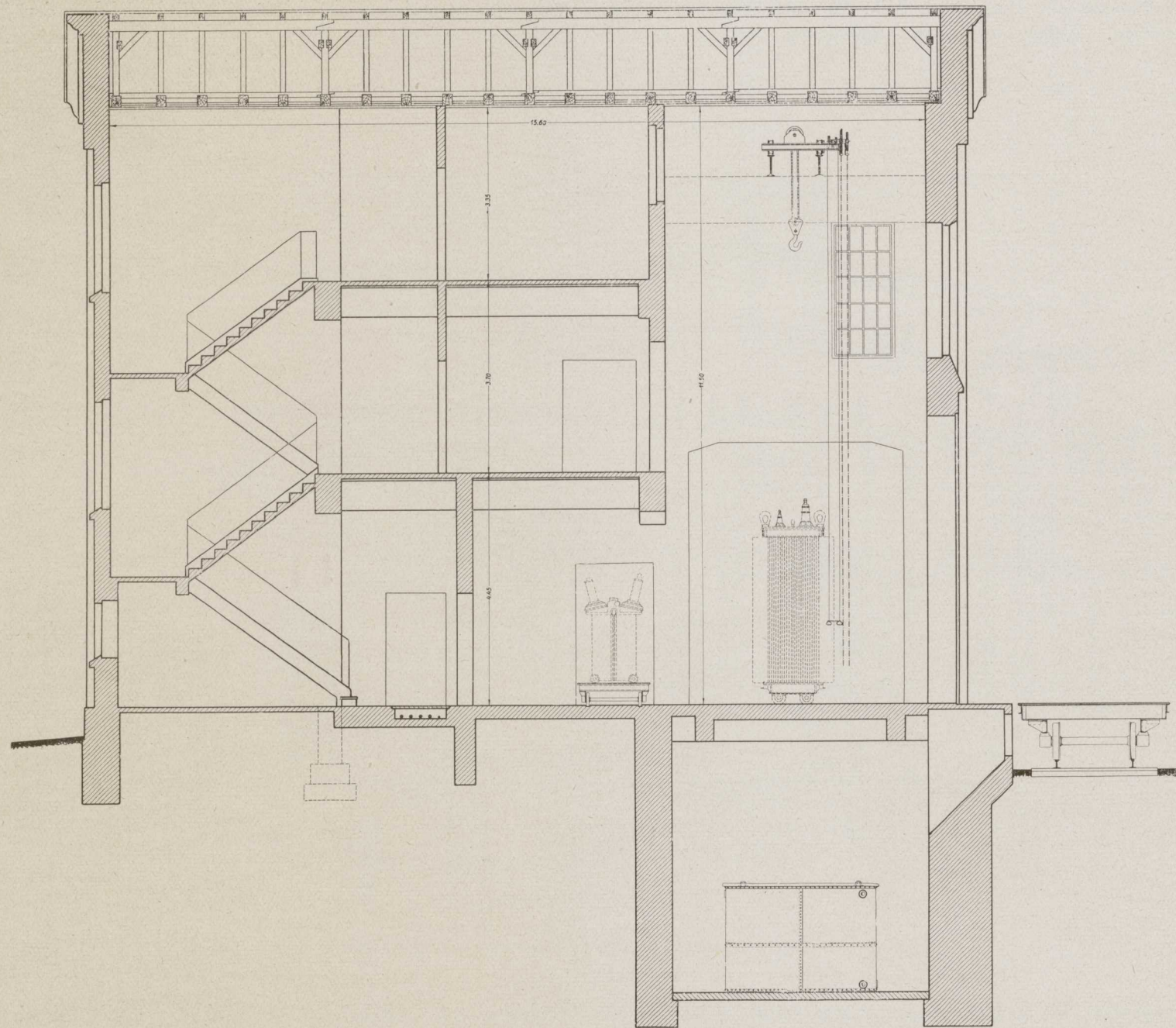
Abbildung 54: Umspannwerk Steyr, Querschnitt durch Werkstättenraum
