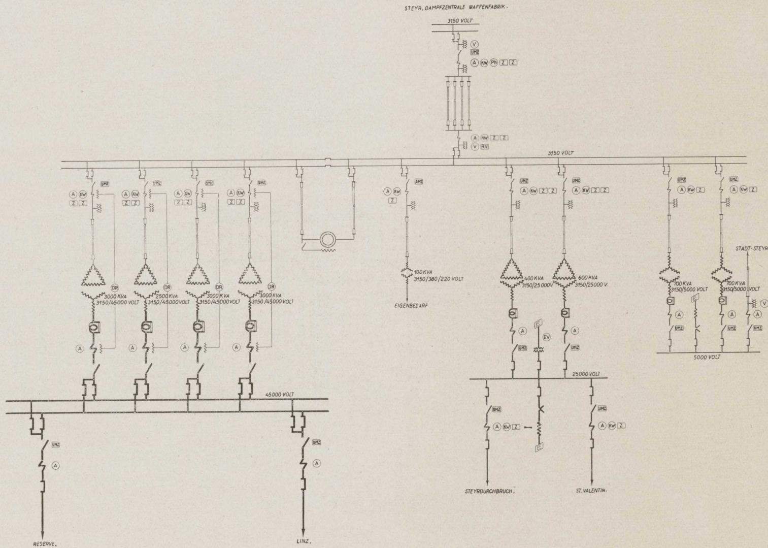
Abbildung 51: Umspannwerk Steyr, Schaltbild
