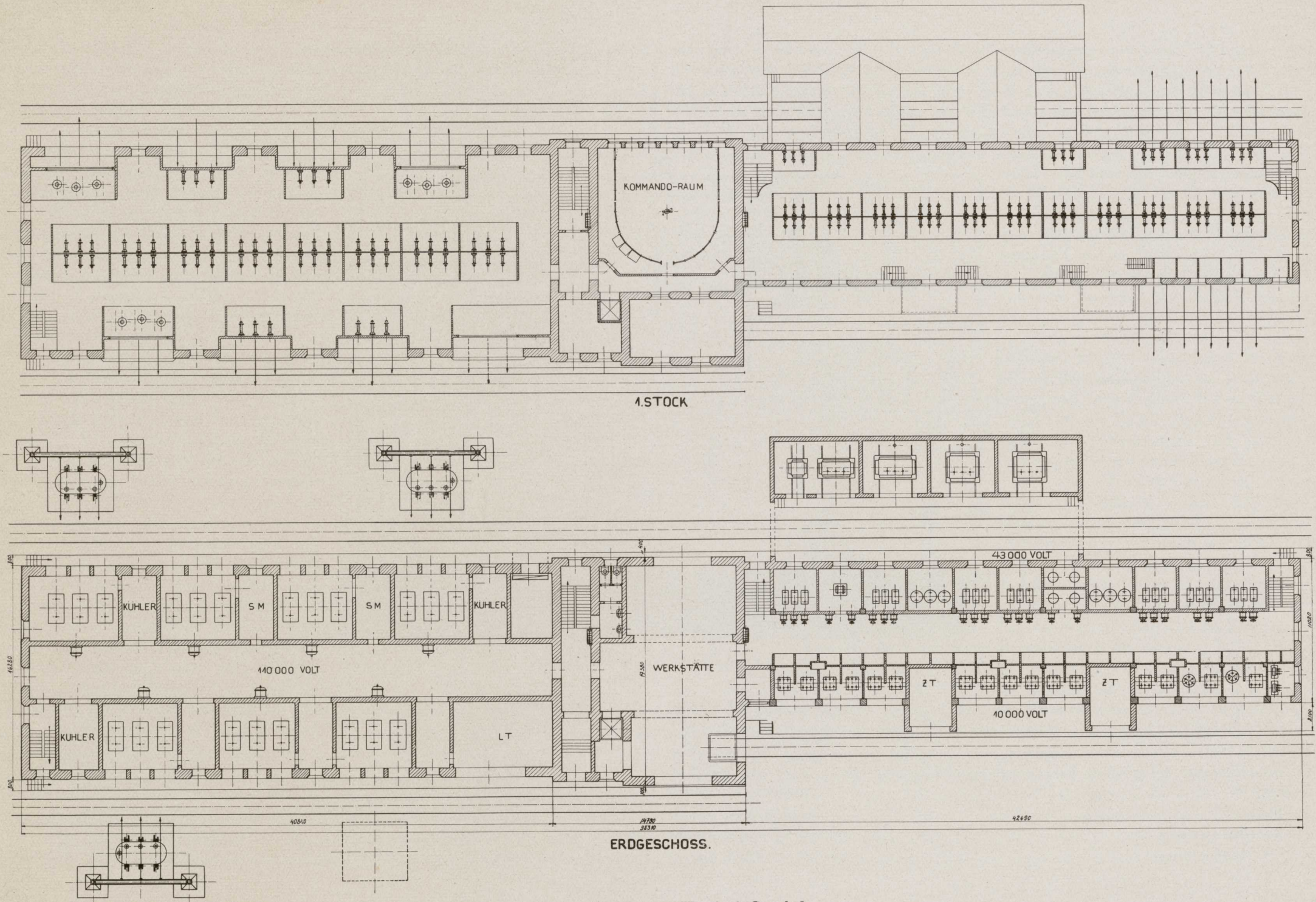
Abbildung 46: Umspannwerk Wegscheid, Grundriß
