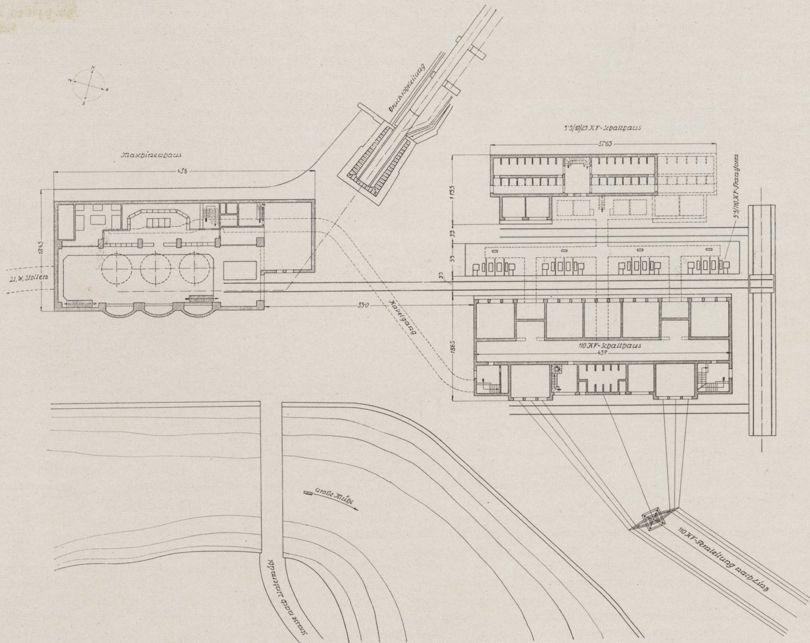
Abbildung 34: Gesamtsituation des Kraftwerkes Fartenstein
