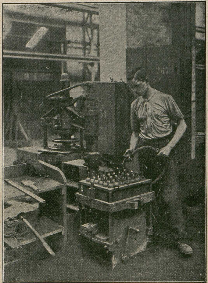
Die gegossenen Handgranaten werden mittels Luftpumpen vom letzten Staub befreit.
