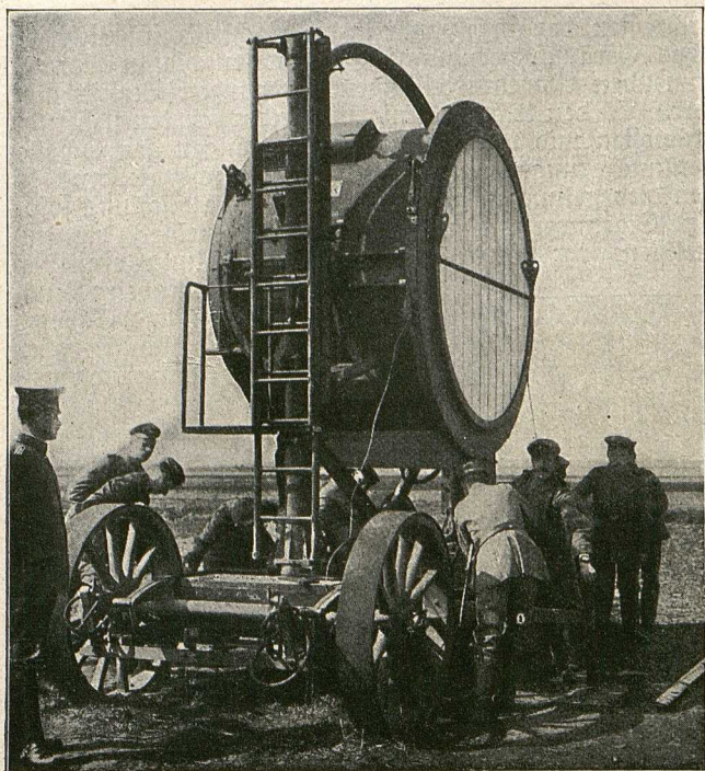
Flak-Scheinwerfer mit 2 Meter Durchmesser und 6000 Meter Leuchtweite.
