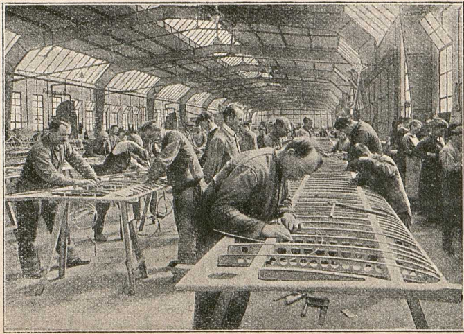
In einer Flugzeugfabrik: Verspannarbeiten an Gerippen von Tragflächen.
