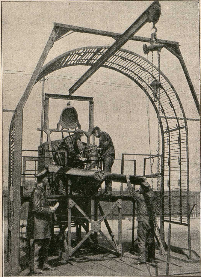
In einer Motorenfabrik: Prüfstand für Flugzeugmotoren, auf dem die Motore vor dem Einbauen in die Flugzeuge einer tagelangen Prüfung unterzogen werden. Der Prüfstand ist mit einem Witter umgeben, das abprallende Propellererteile auffangen soll.
