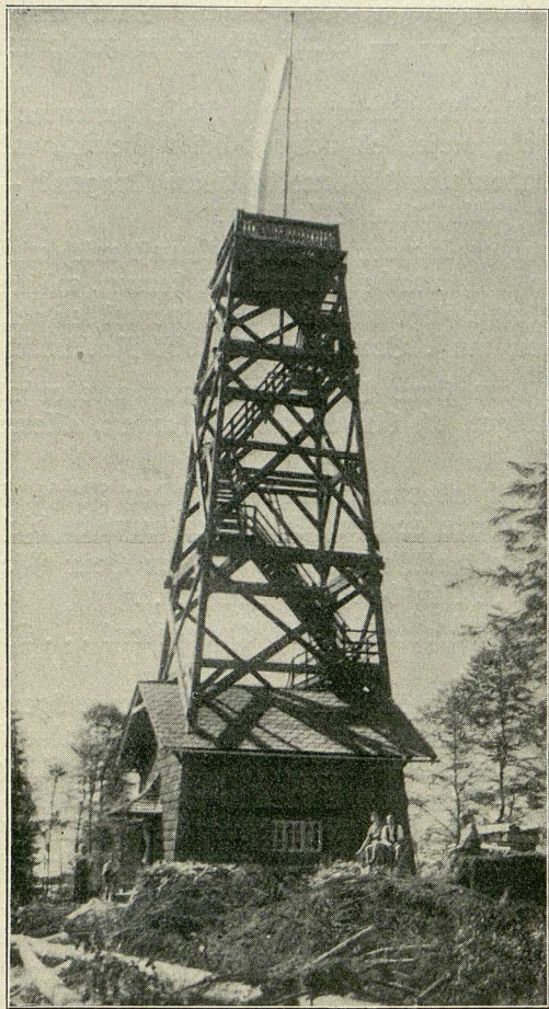
Die Jubiläumswarte auf dem Grünberg bei Gmunden neuerbaut von der Sektion Gmunden des Ost. Touristenklubs.
