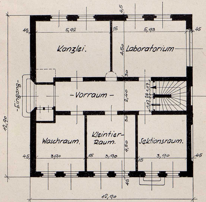
24. Grundriß.
