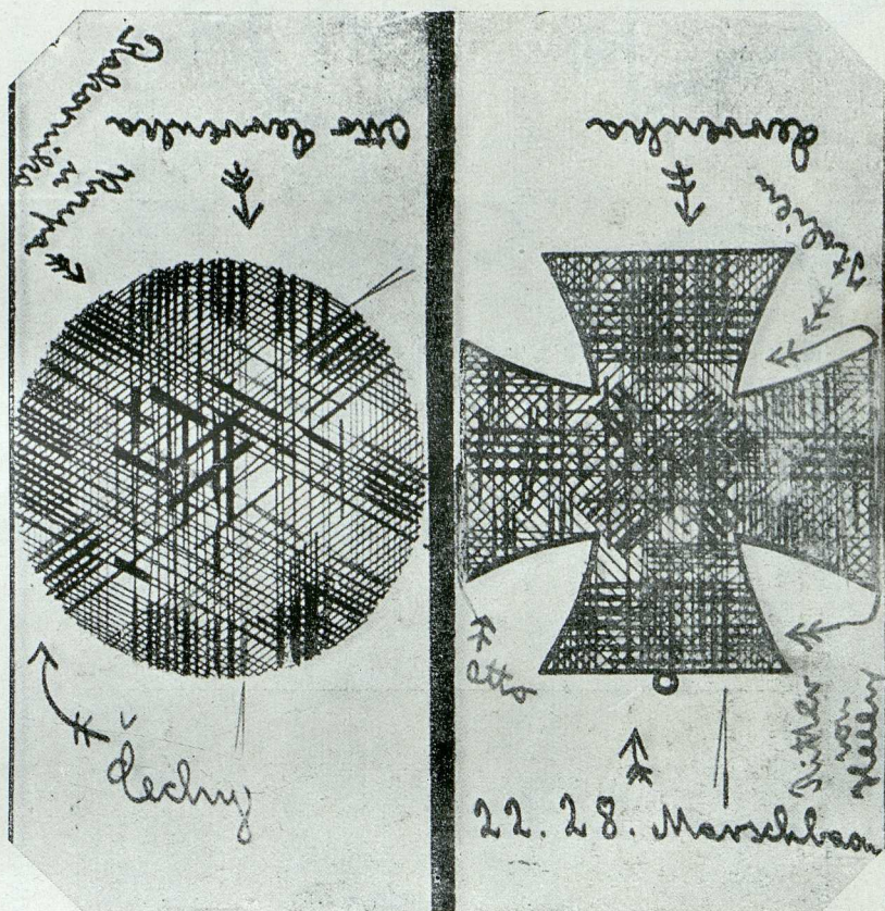
Chiffrierte Nachrichten.
