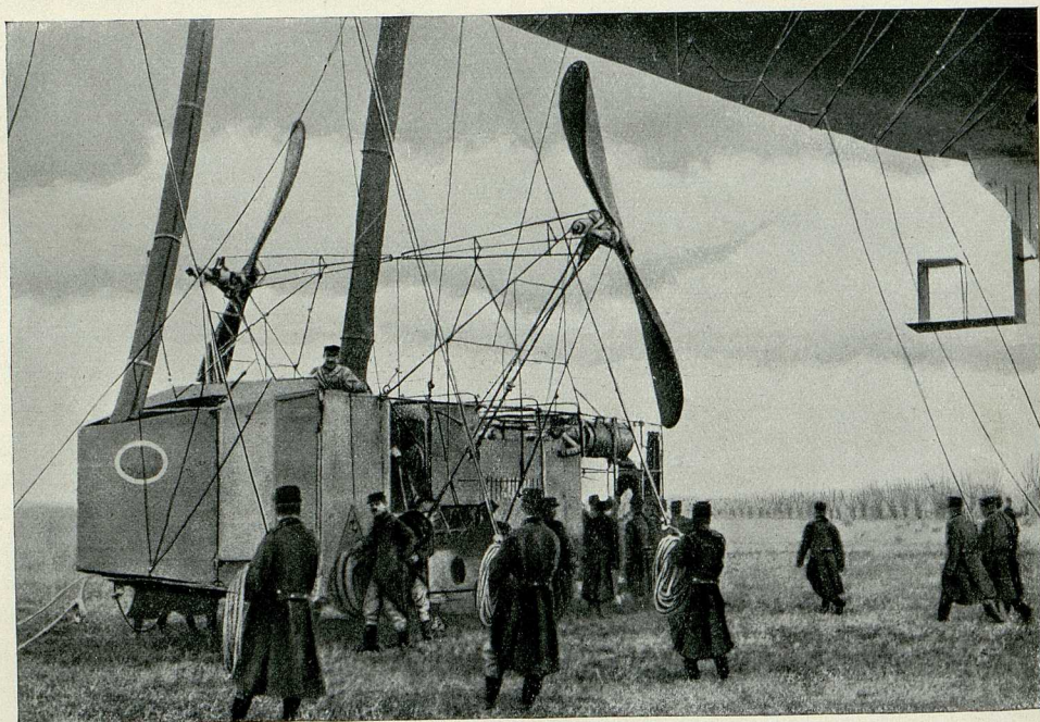
Die gepanzerte Gondel eines französischen lenkbaren Luftschiffs
