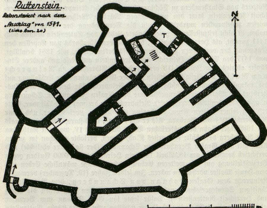
2. Grundriß des Schlosses Rutenstein.
