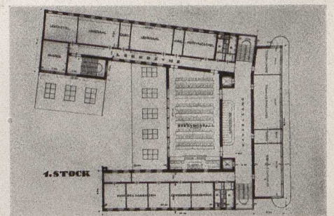
Hauptgrundriß
