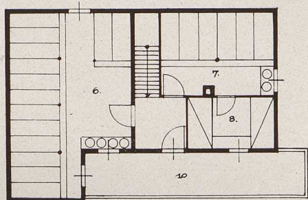
Jahnheim Kirchsclag. 1932 Grundriß und Schnitt
