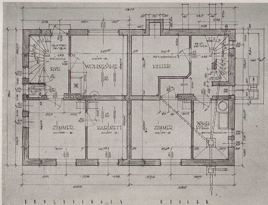
Grundrisse zu obigem Doppelwohnhaus. 1926
