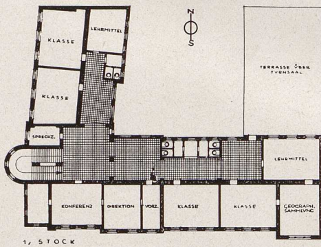
Mädchenlyzeum in Linz, Grundriß
