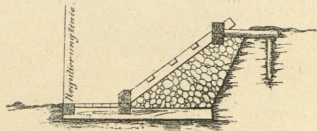
Fig. 131. Querschnitt.
