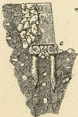
Fig. 130. Querschnitt.
