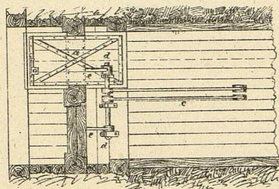
Fig. 120. Grundriss.
