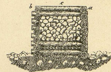
Fig. 128. Querschnitt.
