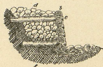
Fig. 127. Querschnitt.
