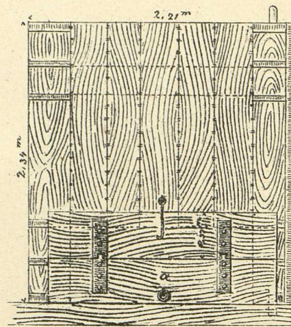
Fig. 113. Ansicht.
