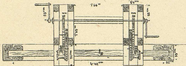
Fig. 111. Grundriss.
