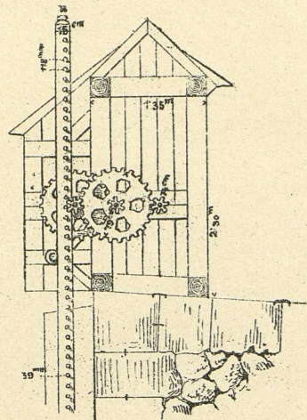
Fig. 111. Querschnitt.
