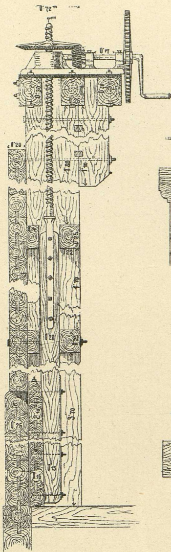
Fig. 110 c. Querschnitt.
