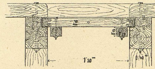
Grundriss des Thores.
