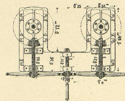
Grundriss der Hebevorrichtung.
