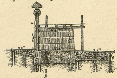
Fig. 84. Querschnitt.
