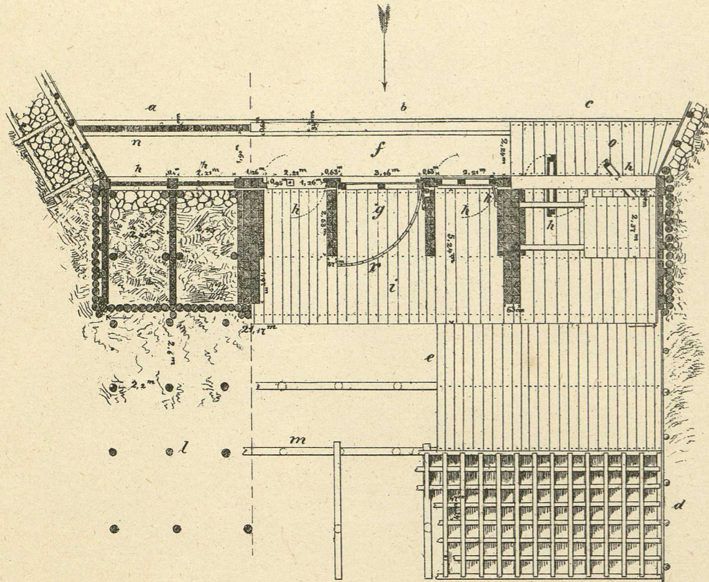
Fig. 82. Grundriss.
