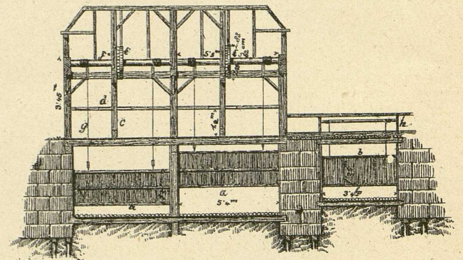
Fig. 84. Querschnitt.
