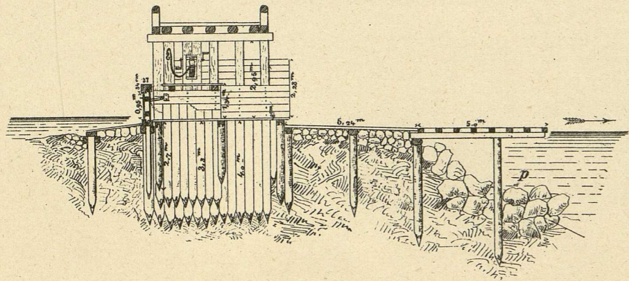
Fig. 82. Querschnitt.
