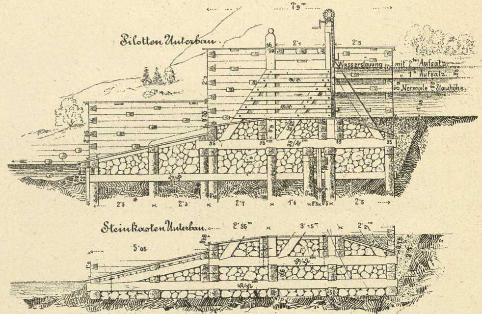
Fig. 83. Längenschnitt.
