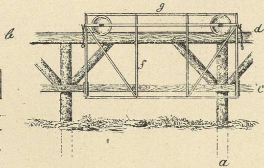
Fig. 71. Querschnitt.
