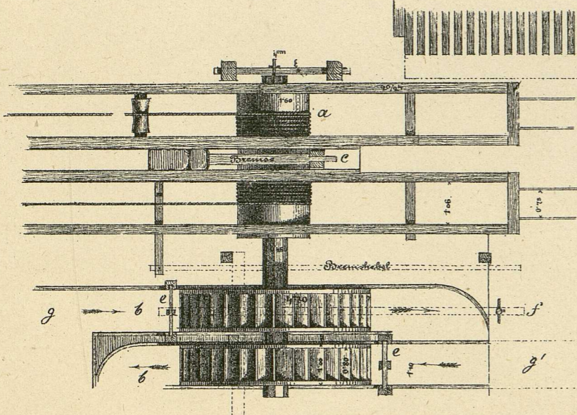
Fig. 72. Grundriss.
