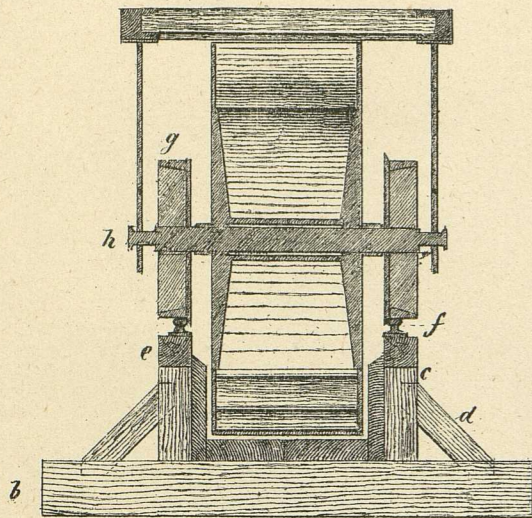
Fig. 69. Querschnitt.
