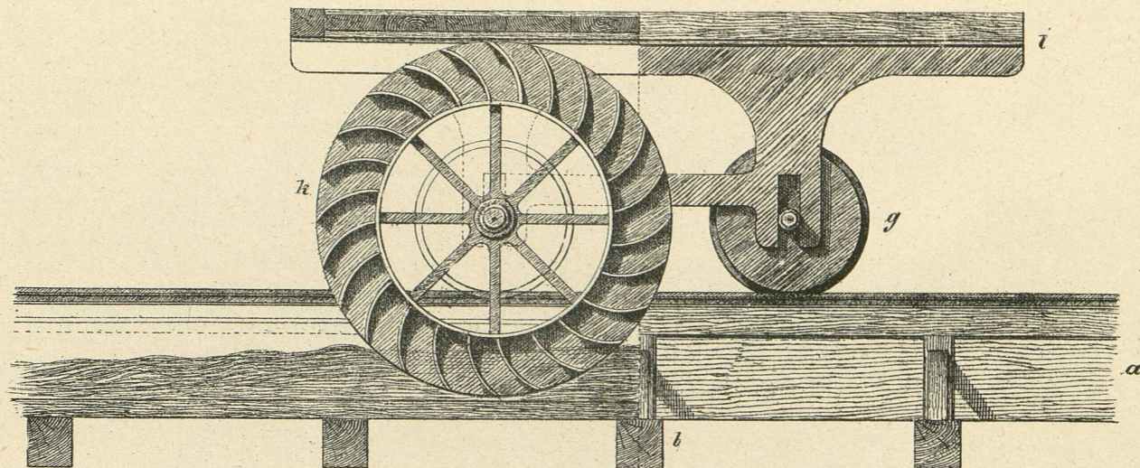
Fig. 69. Längenschnitt.
