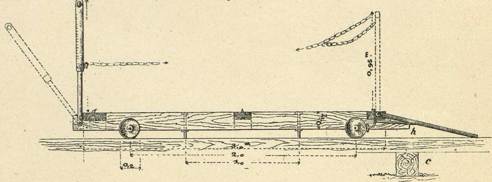
Fig. 70. Längenschnitt.
