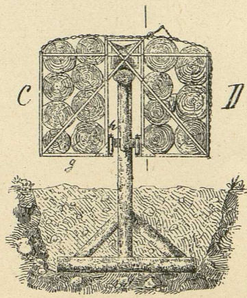
Fig. 71. Querschnitt.
