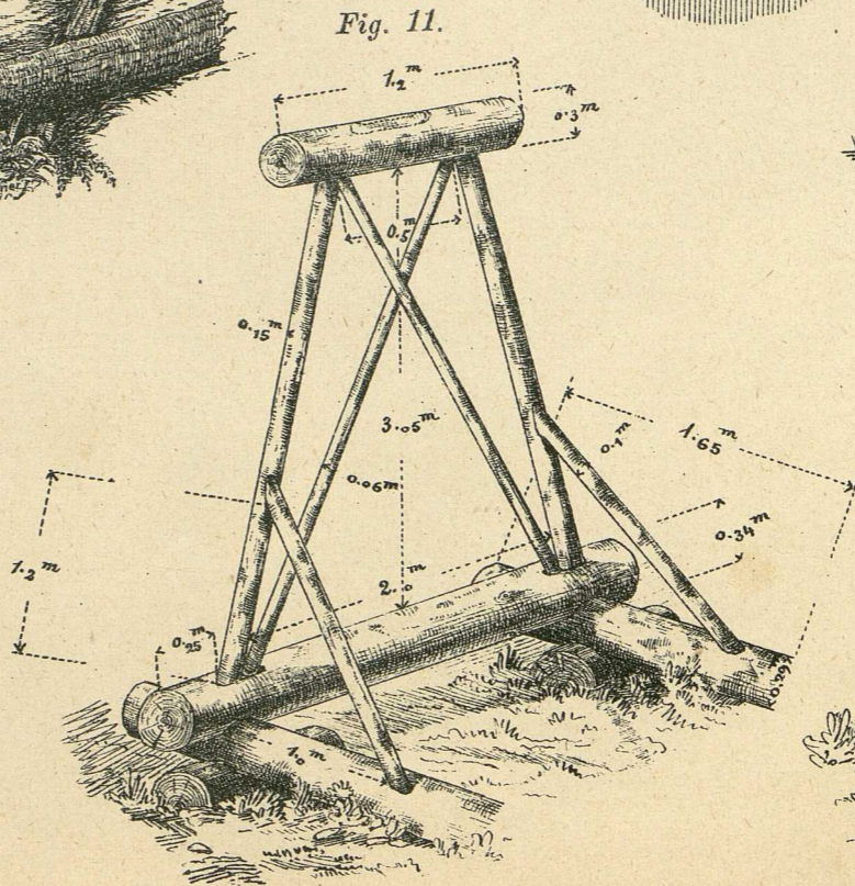
B. Halbkastenjoch.
