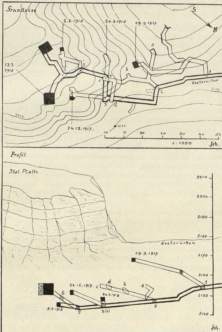
Österreichisches Stollensystem unter der ital. Platte.
