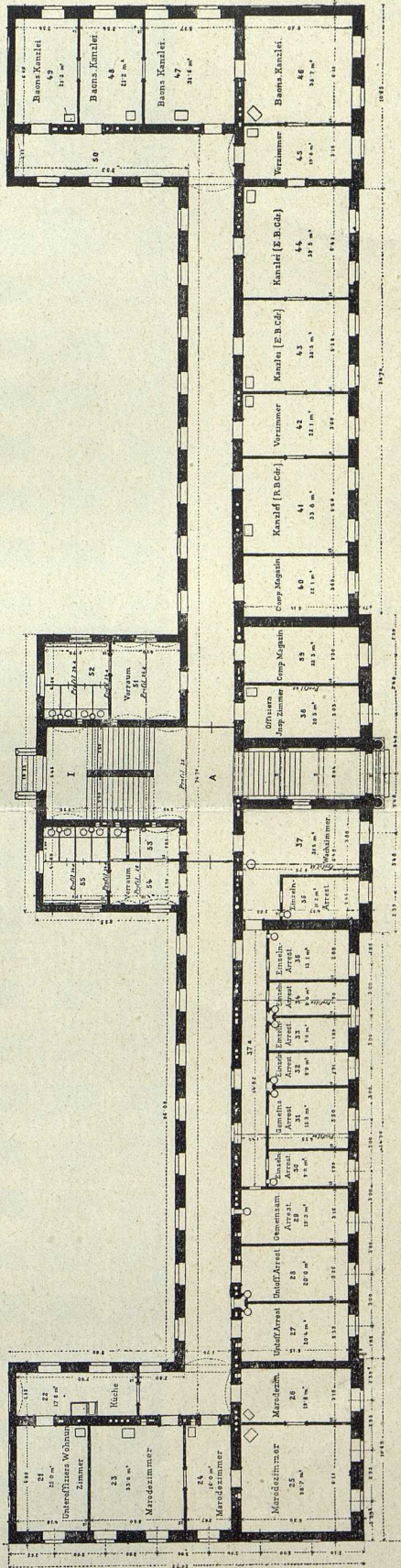
Grundriss vom Erdgeschoss.
