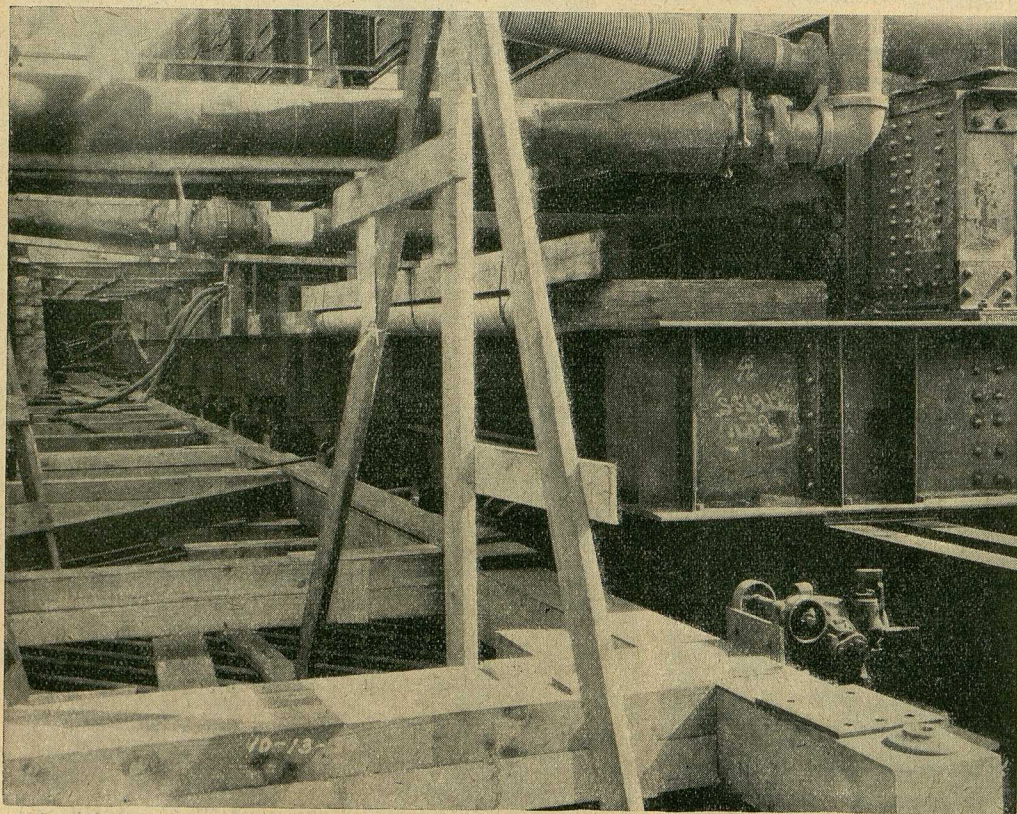
Damit der Betrieb weitergeht, werden Leitungen und Kanäle mit beweglichen Anschlüssen versehen
