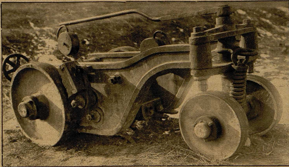
Maschinen, welche die Russen auf ihrem Rückzuge zum Auf- reißen und Unwegbar- machen der Chausseen benutzten.
