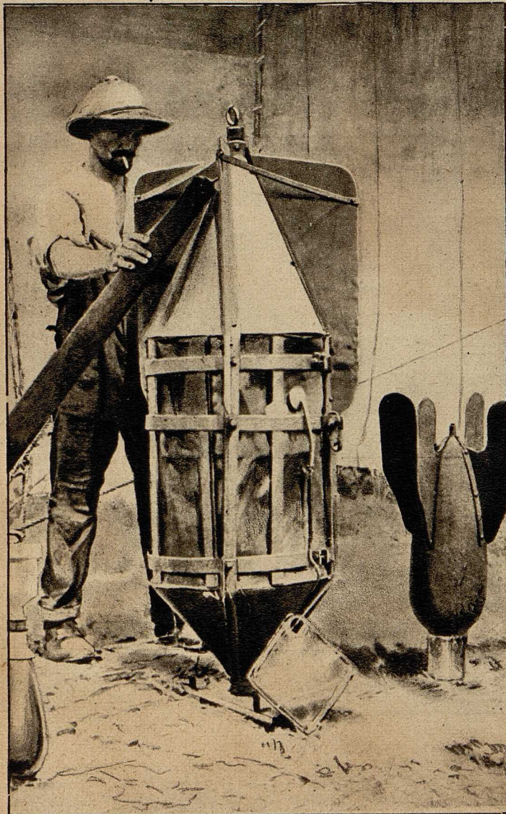
Eine eigenartige Fliegerbombe, die jetzt von französischen Fliegern erprobt wird, und von der sich die Franzosen große Wirkungen versprechen. (Vereinigete Fotob.)
