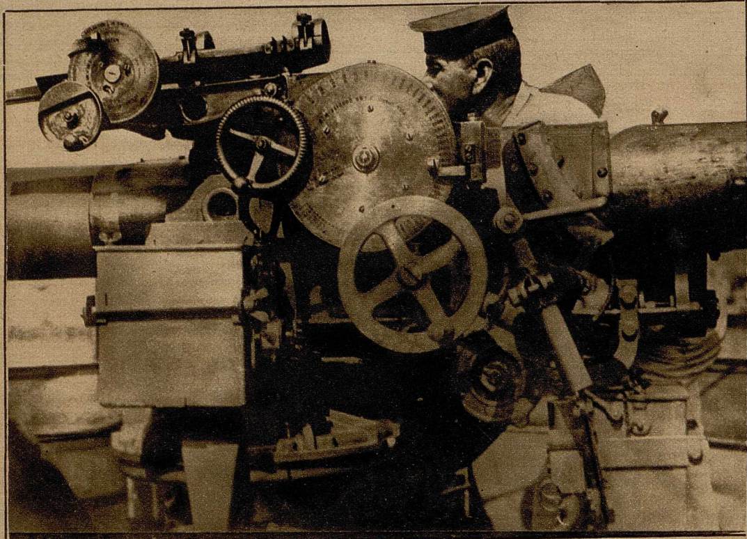
Nebenstehendes Bild: Die Richt- und Zielvorrichtung einer Schiffs- kanone an Bord eines englischen Dreadnoughts. (Phot. B. I. G.)
