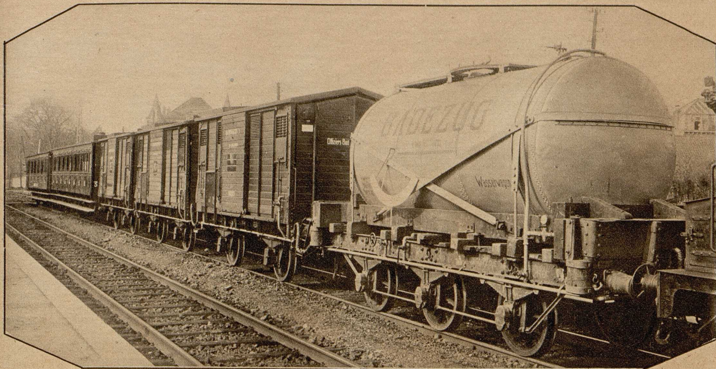
Der Wasserwagen, die Bade- und Ankleidewagen und der Wohnwagen des Badezuges beim 1. Bayerischen Reserve-Korps. (Phot. Brämer.)
