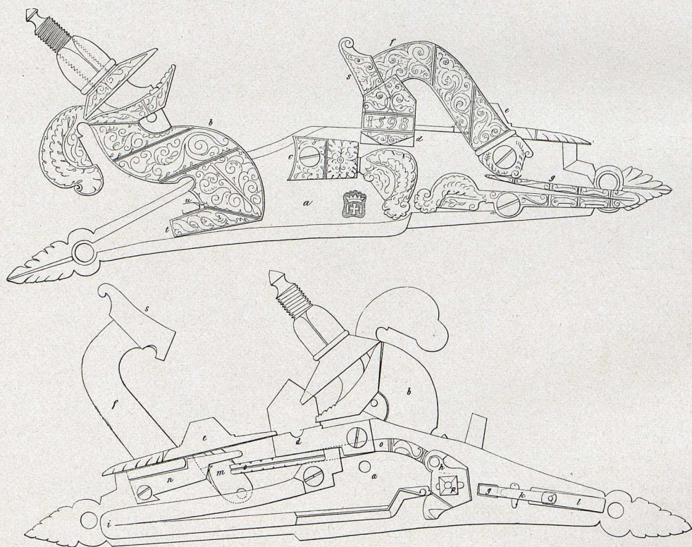
Bild 91. Das holländische Batteriesteinschloß (Schnapphahnschloß) mit 14 Teilen, um 1500 Beim spanischen Schnapphahnschloß sind alle Teile außen, beim holländischen innen, beim holländischen aber Nachteil: keine Ruhrast
