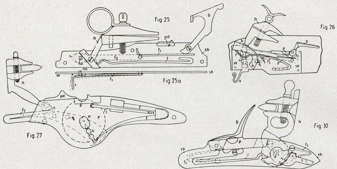
Fig. 25. Steinschloß, etwa 1500—1520. Fig. 25a. Anordnung der Stange und Stangenfeder. Fig. 26. Steinschloß mit Batterie und zwei Rasten, etwa 1620—1640. Fig. 27. Radschloß, etwa 1520—1540. Fig. 30. Steinschloß, etwa 1640—1660. Aus K. Maleyka, Aus der Vorzeit unserer Jagdgewehre (1938)
