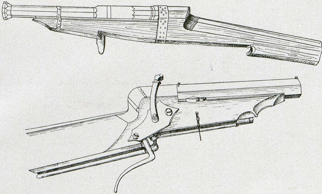
Bild 88. Hakenbüchse und Handbüchse mit Luntenschloß
