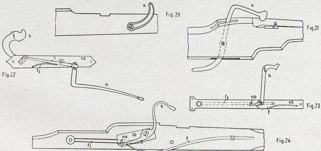
Bild 89. Das Schloß, zeitliche Entwicklung
