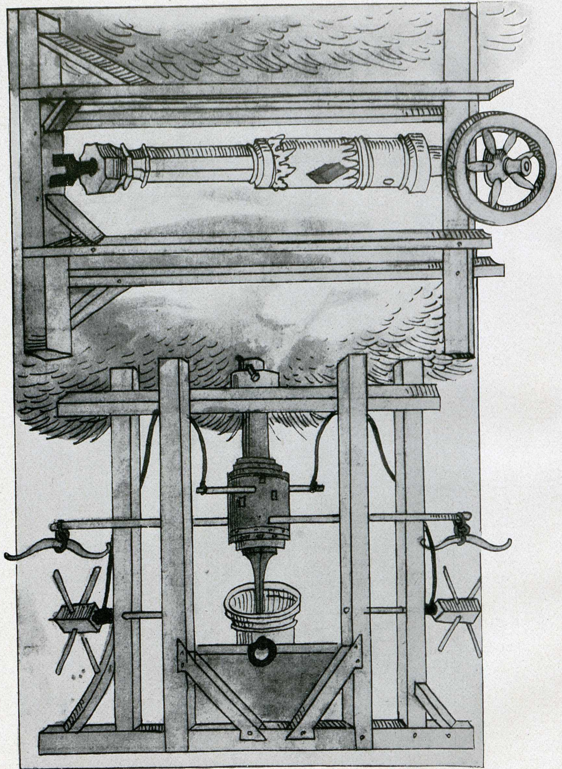
Bild 70. Geschützbohrmaschine. Oben: bohrt von unten nach oben (um 90° gedreht gedacht)
