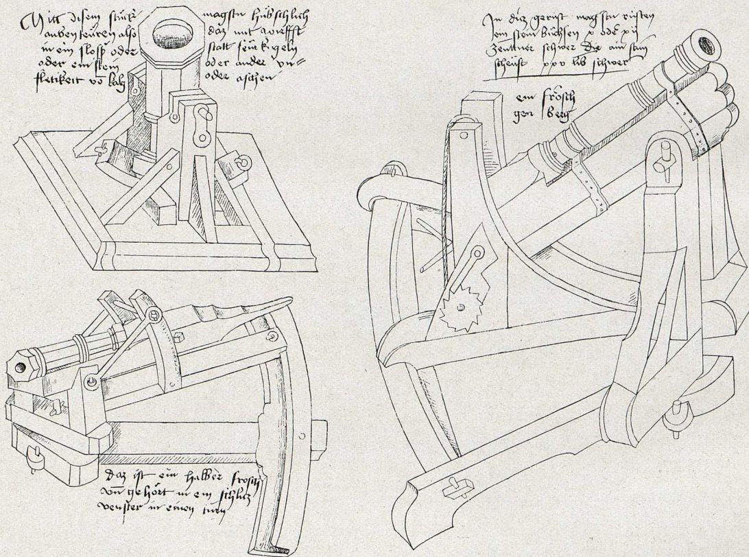
Bild 57. Hochgebautes Lager mit Seiten- und Höheneinstellung
