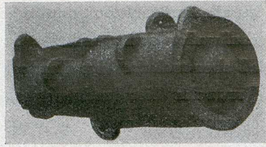
Rechts: Steinbüchse aus Pößneck i. Thür.
