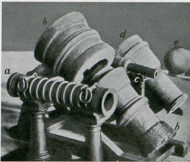
Bild 48. Bombarden aus dem 14. u. 15. Jahrhundert, Zeughaus Berlin
