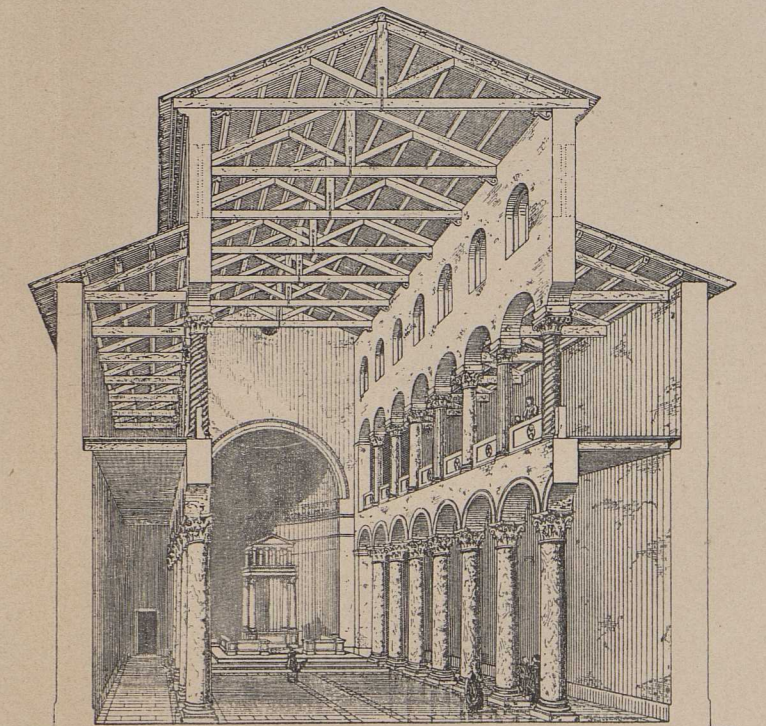
5b. Basilikenbau [S. 790].
