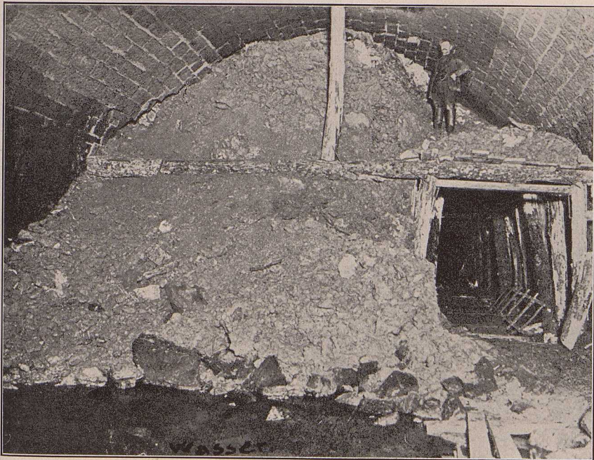
Bild 15. Sprengstelle im Innern des Tunnels bei Montmédy mit einem der durchgetriebenen Sohlstollen. (Zu Seite 78)
