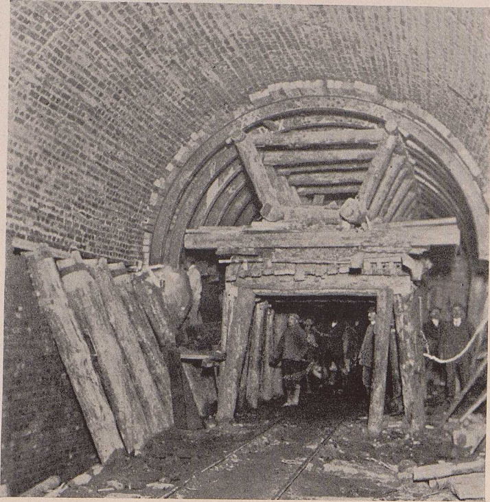
Bild 14. Wiederherstellungsarbeiten am Tunnel bei Trois-Ponts. (Zu Seite 75.)
