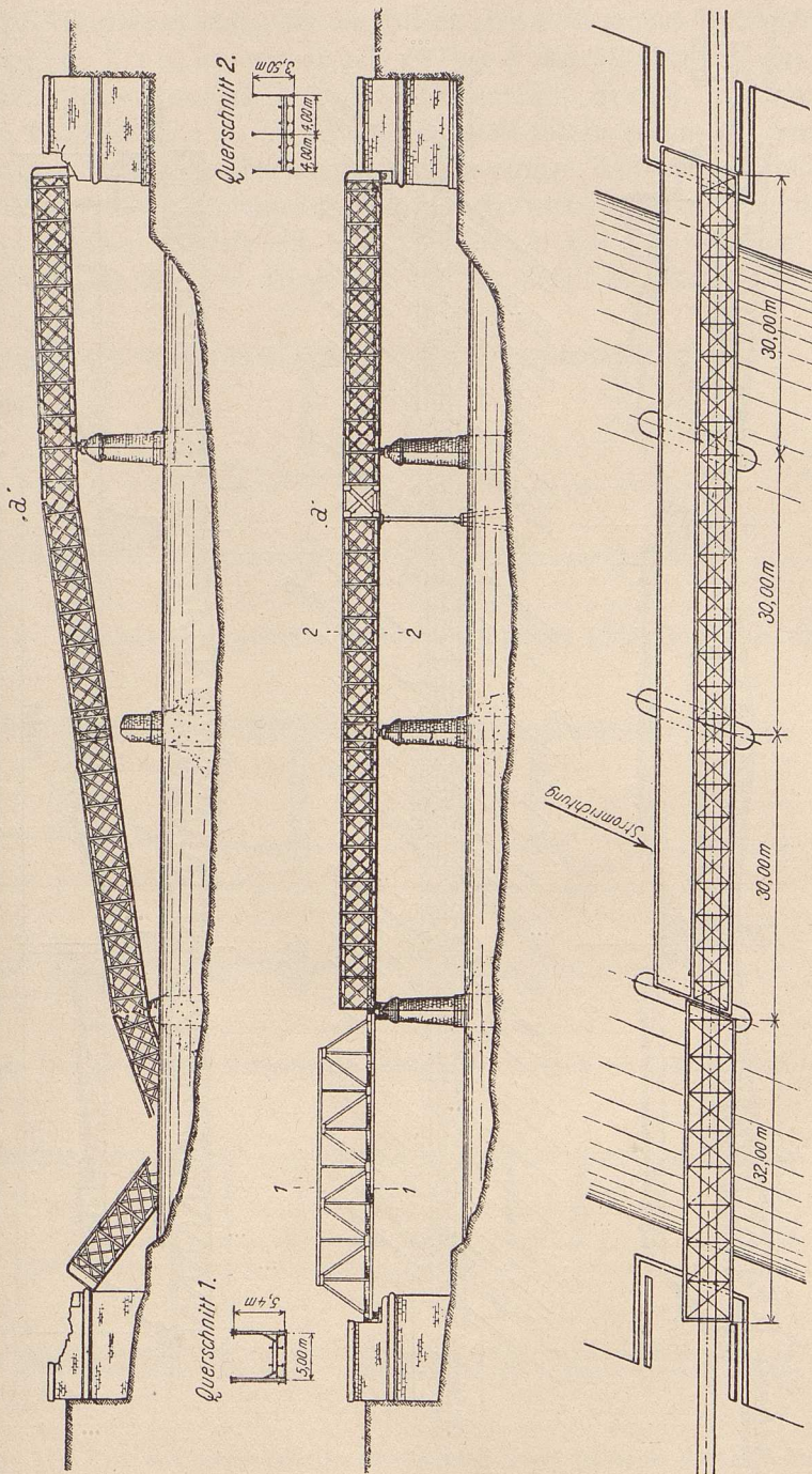
Stigge 7. Die geförte und wiederhergestellte Maas-Brücke bei Anhee.
