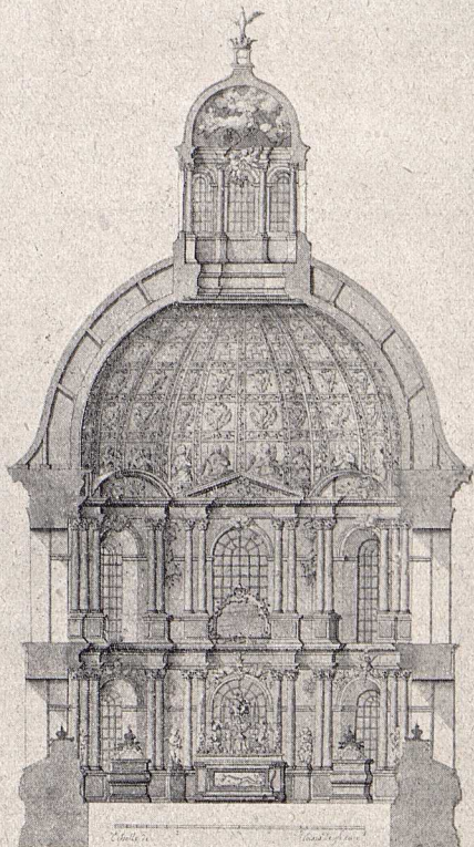
Il Palazzo Imperiale di Napoli, veduta della cupola, e dell'interno. Disegnata da G. B. Piranesi, e incisa da G. G. B. Piranesi. Roma, 1763.
