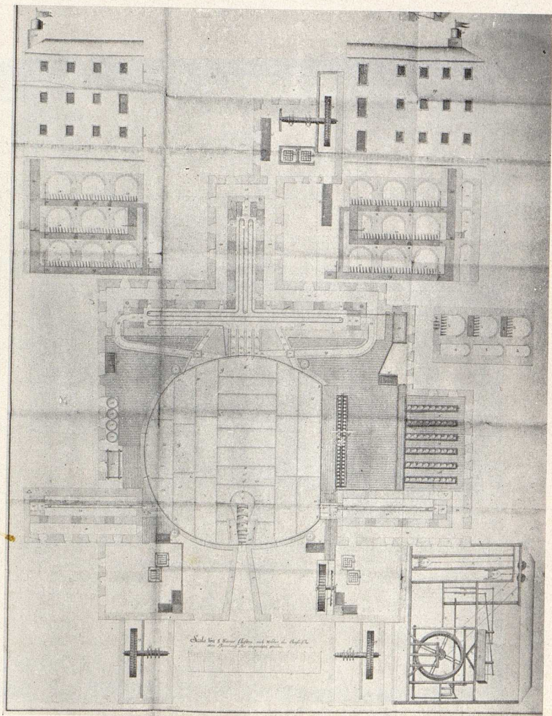
Fig. 13. Oberes Sudhaus in Ebensee, Pfanne, 1765.
