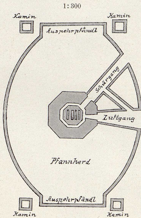
Fig. 7a. Schematische Darstellung der Sudanlage nach Dr. Lebzelter.
