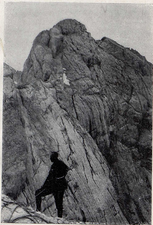
Abb. 19. Rillen und Kluffarren an der Schneebergwand.
